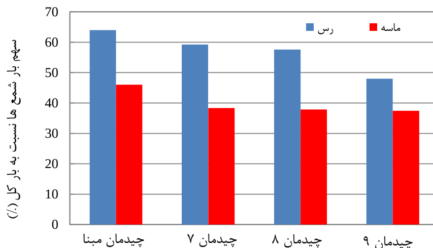
شکل ۲۰: سهم بارگیری شمع‌ها نسبت به بار کل
