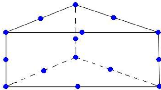
شکل ۴: المان منشوری ۱۵ گرهی
