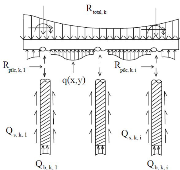
شکل ۱: اندرکنش بین شمع، خاک و پی [۱۳]
