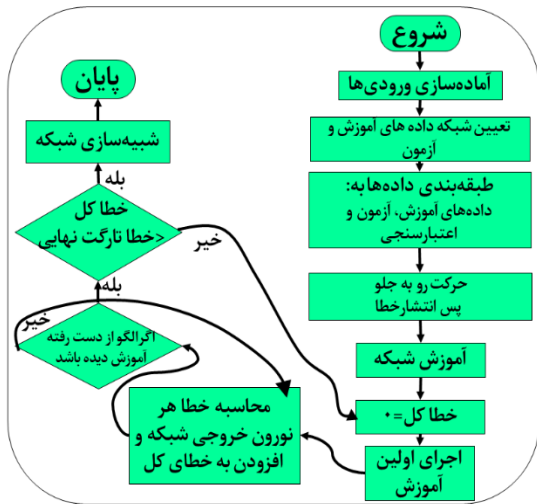
شکل ۵: نمودار سازوکار شبکه‌های عصبی مصنوعی [۱۹].
