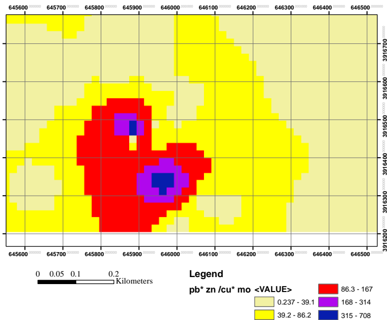
شکل ۷: نحوه توزیع و مقادیر شاخص زونالیت‌ها برای کانی‌سازی تپ مس پورفیری در منطقه
