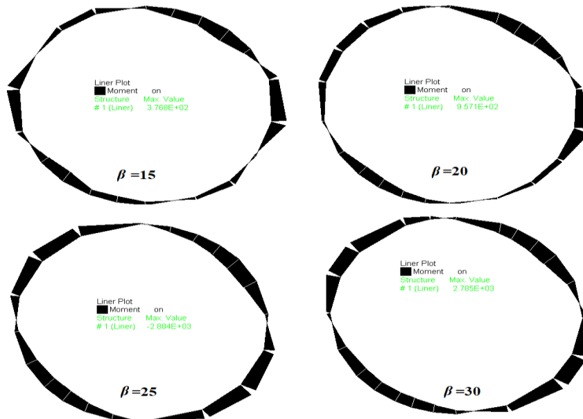
شکل ۱۸: کانتور ممان خمشی (N.m) القایی در سطح مقطع لوله برای حالت‌های مختلف زاویه شیروانی نامحدود ناشی از تغییر شکل‌های بیضوی ایجاد شده در مقطع لوله به وسیله‌ی بار زمین لرزه.
