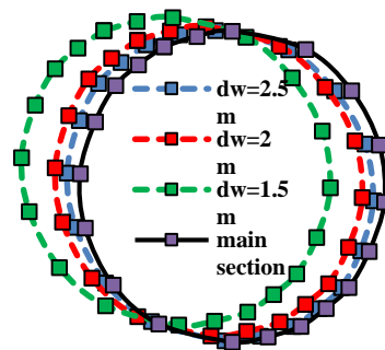
شکل ۹: تغییرات مکانی سطح مقطع لوله تحت بار زمین لرزه برای حالت‌های مختلف سطح آب زیرزمینی.
