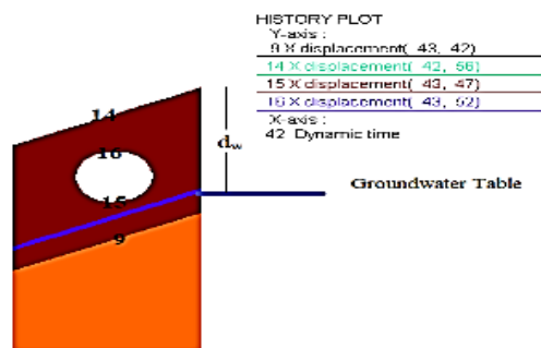
شکل ۸: تاریخچه جابجایی نقاط مختلف لوله مدفون و لایه خاکی با شیروانی نامحدود (بر حسب متر و ثانیه).
