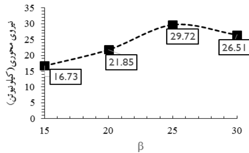
شکل ۱۶: نمودار نیروی محوری القایی در سطح مقطع لوله نسبت به زاویه شیروانی خاکی نامحدود.
