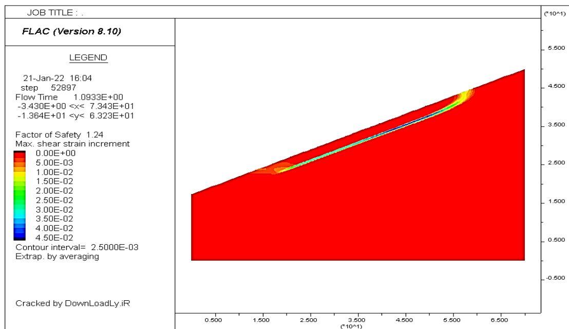
شکل ۶: مقادیر فاکتور ایمنی و کرنش برشی محاسبه‌شده
