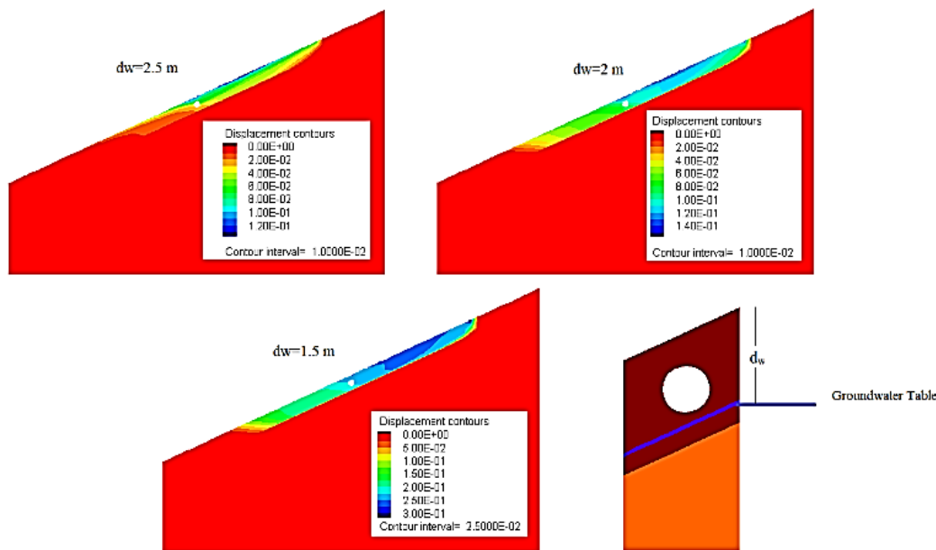
شکل ۷: جابجایی‌های لایه خاکی با شیروانی نامحدود برای حالت‌های مختلف dw (بر حسب متر).
