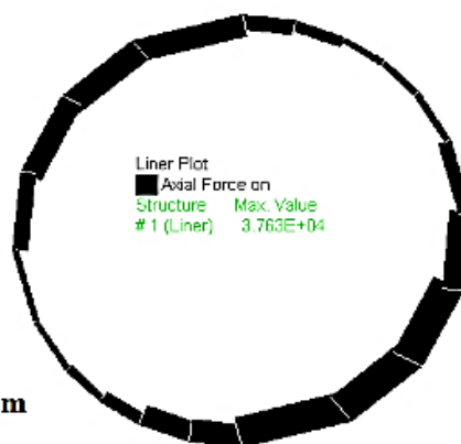
شکل ۱۰: کانتور مقادیر ممان (N.m) و نیروی محوری (N) القاشده در سطح مقطع لوله.
