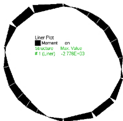
شکل ۱۰: کانتور مقادیر ممان (N.m) و نیروی محوری (N) القاشده در سطح مقطع لوله.
