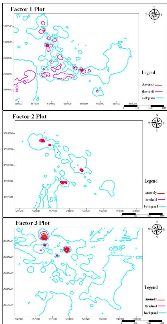
شکل ۱۰: نقشه ژئوشیمیایی فاکتور ۱، ۲ و ۳ با روش فرکتال
