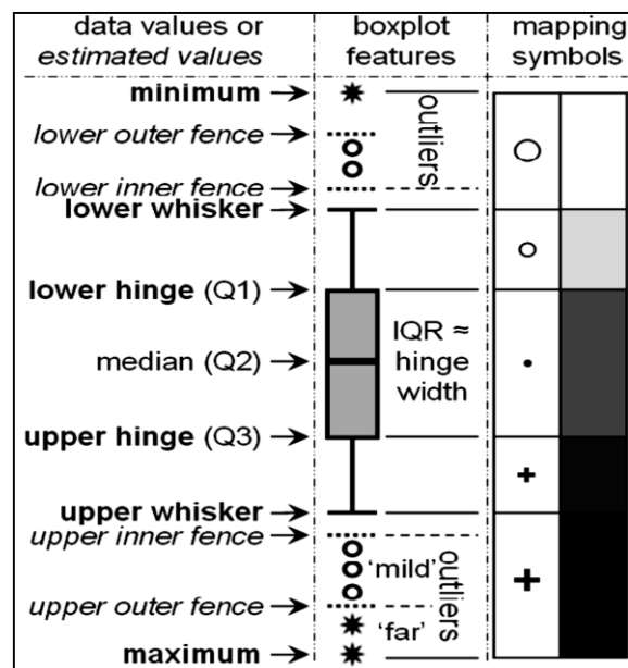
شکل ۱۱: علائم نمودار جعبه‌ای و کلاس‌بندی داده‌ها [۱۱]
