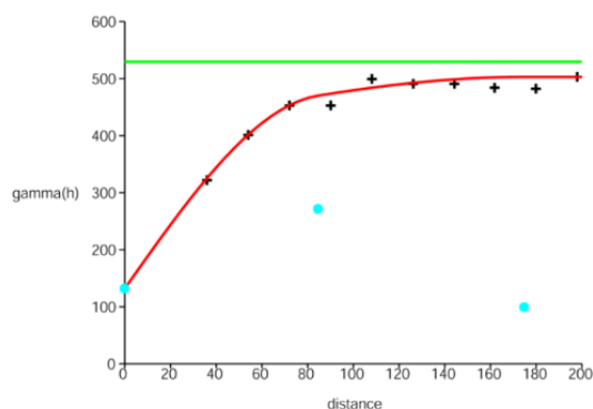
شکل ۱۴: برازش مدل به واریوگرام برای رنگ آبی با گام 18 متری
