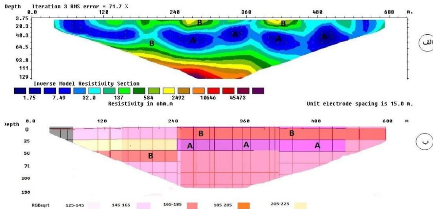
شکل ۲۴: نقشه هم مقاومت ظاهری پروفیل استو پایل CC و مقطع سیستم رنگ I_{rgb} [۸]
