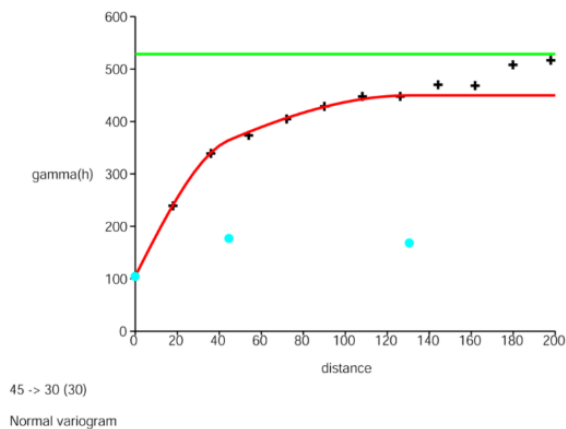
شکل ۱۲: برازش مدل به واریوگرام برای رنگ قرمز (R) با گام ۱۸ متری
