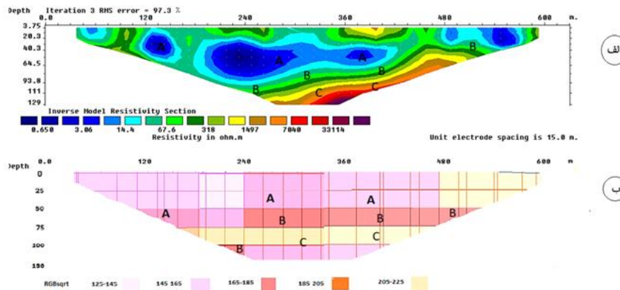
شکل ۲۵: نقشه هم مقاومت ظاهری پروفیل شمالی DD و مقطع سیستم رنگ Irgb (الف)
