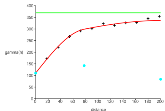
شکل ۱۳: برازش مدل به واریوگرام برای رنگ سبز با گام 18 متری
