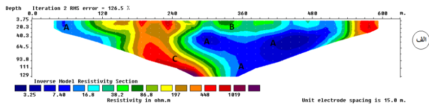
شکل ۲۲: نقشه هم مقاومت ظاهری پروفیل غربی AA و مقطع سیستم رنگ I_{rgb} [۸]
