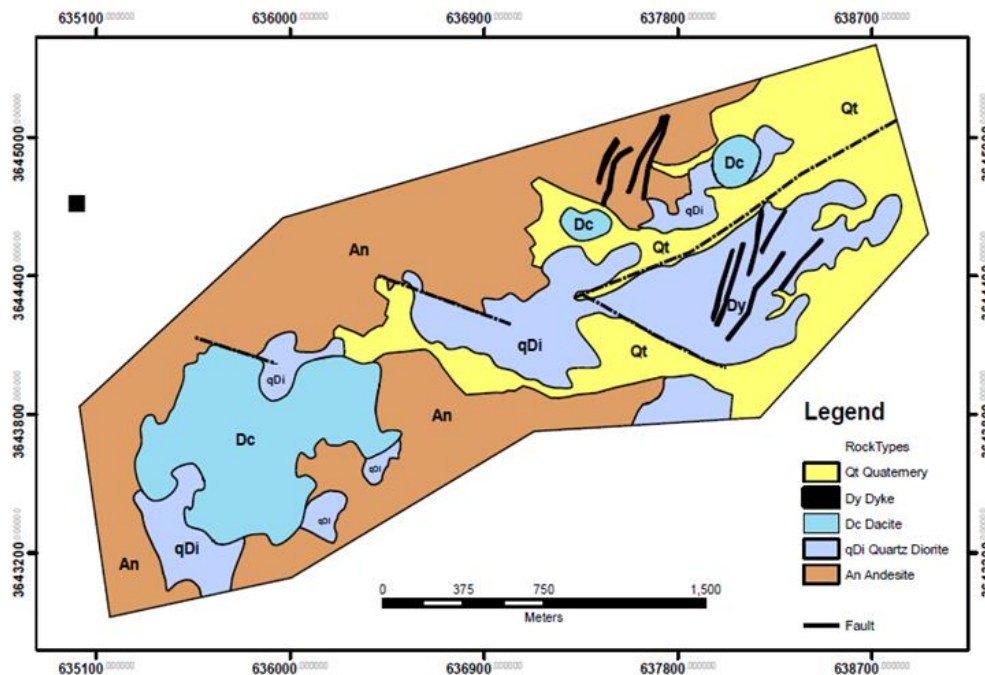
شکل ۴: نقشه زمین‌شناسی کانسار مس پورفیبری کهنگ (مقیاس ۱:۱۰۰۰۰) [۴]
