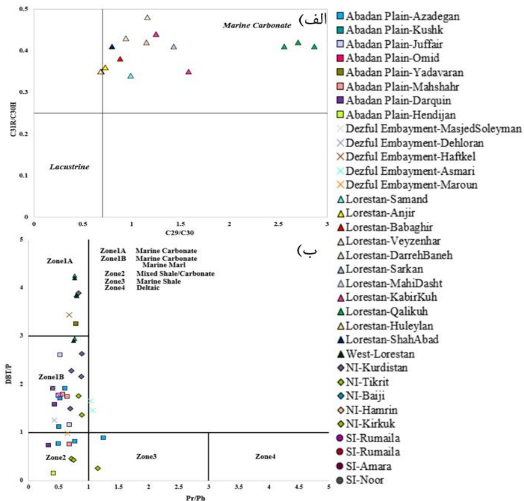
شکل ۴: الف) نمودار نسبت C31R/C30h به C29/C30 نشان‌دهنده‌ی محیط رسوب‌گذاری (دریایی، خشکی، باتلاقی یا دلتایی) است [۳۷]. ب) نسبت DBT/P در مقابل Pr/Ph که نمایانگر محیط رسوب‌گذاری سنگ مادر مورد مطالعه است.
