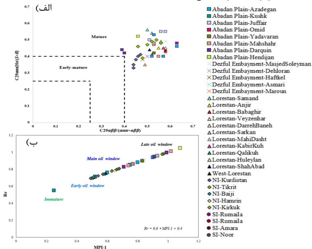
شکل ۵: الف) نمودار نسبت C29aaa20S/(20S+20R) به C29a\beta\beta/(aaa+a\beta\beta) به جهت تخمین میزان بلوغ نمونه‌های مورد مطالعه [۳۶]. ب) نمودار نسبت MPI-1/Rr نشان‌دهنده بلوغ حرارتی در نمونه‌های مورد مطالعه است.
