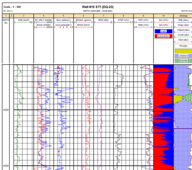
شکل ۴: ستون پنجم، نگار ضریب سیمان‌شدگی محاسبه شده با استفاده از نگار چگالی است
