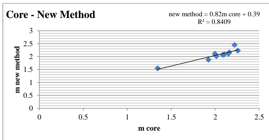
شکل ۵: مقایسه نتایج به دست آمده با مقادیر ضریب سیمان‌شدگی حاصل از آزمایشات مغزه
