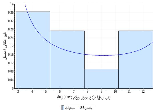
شکل ۹: تابع توزیع احتمال جانسون SB ضریب عکس‌العمل بستر در تنش جانبی ۳ کیلوگرم بر سانتی‌مترمربع
