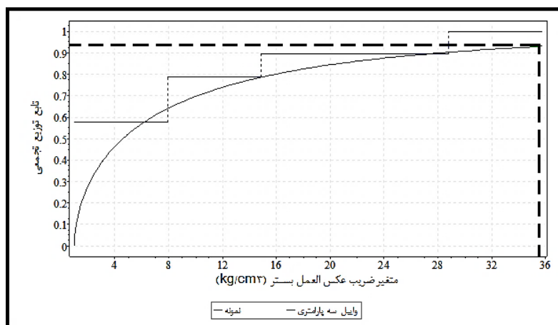
شکل ۱۳: تابع توزیع تجمعی وایبول در تنش جانبی ۰/۷ کیلوگرم بر سانتی متر مربع
