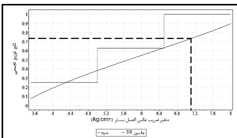
شکل ۱۶: تابع توزیع تجمعی جانشون SB برای آزمایش بارگذاری صفحه‌ای (در تنش جانبی تقریباً صفر)
