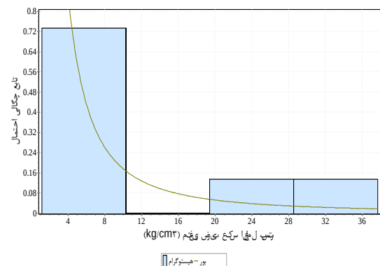
شکل ۷: تابع توزیع احتمال بور ضریب عکس‌العمل بستر در تنش جانبی ۵/۵ کیلوگرم بر سانتی‌مترمربع
