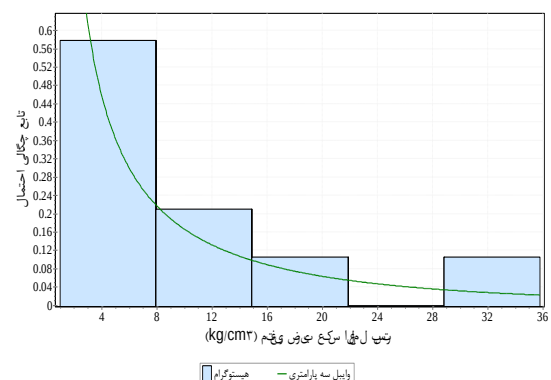
شکل ۸: تابع توزیع احتمال ویبول ضریب عکس‌العمل بستر در تنش جانبی ۷/۰ کیلوگرم بر سانتی‌مترمربع
