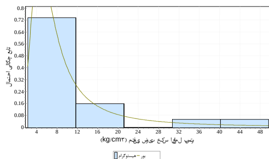
شکل ۱۰: تابع توزیع احتمال بور ضریب عکس‌العمل بستر در تنش جانبی ۴/۲ کیلوگرم بر سانتی‌مترمربع
