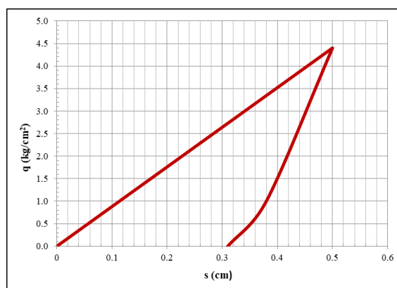
شکل ۴: نمودار فشار- نشست از آزمایش بارگذاری صفحه‌ای صحرایی (یکی از ۸ نقطه)
